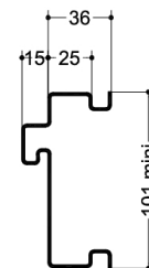
Profil banché
