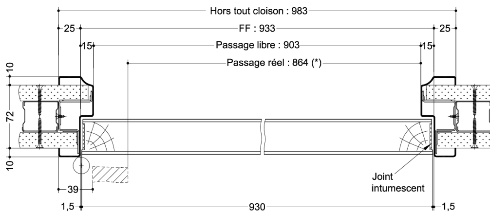
(* unité de passage à respecter selon réglementation et PMR. cf. annexes)
