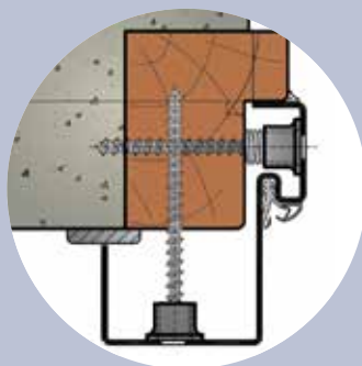
SYSTÈME VÉRINS-ÉCROUS
