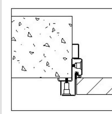
Huisserie Sur Parement
