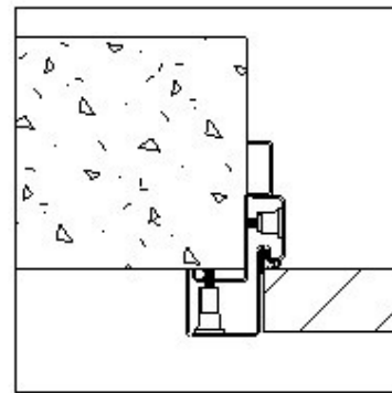
Huisserie Après Parement
