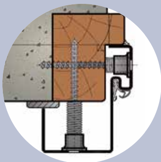
SYSTÈME VÉRINS-VÉRINS*
