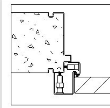
Huisserie Avant Gorge
