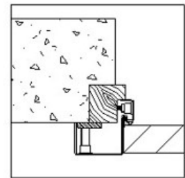
Huisserie Après Chant Plat
