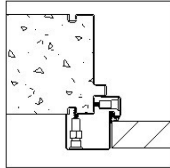
Huisserie Après Gorge
